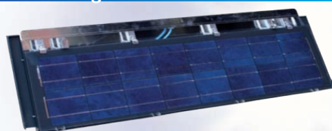
Tuile photovoltaïque Réf. PH PM S'adapte avec des couloirs d'étanchéité en latéral
