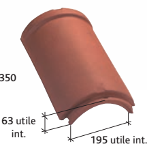
Faitière/arêtier 1/2 rond à emboitement grand modèle (3) (2,5 au ml) Réf. 702. Crochet adapté : crochet F1-Réf. CRP 702
