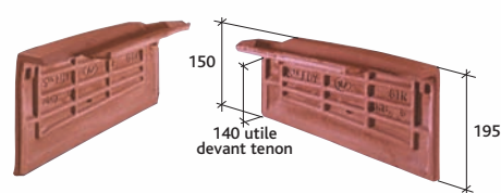
Rive individuelle gauche à emboitement Arboise rectangulaire (2) (4 au ml) Réf.301.40
