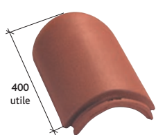
About d'arêtier 1/2 rond (3) à emboitement grand modèle Réf. 851
