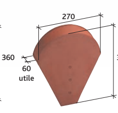
Fronton petit modèle pour faitière 1/2 ronde et faitière conique (petite ouverture) Réf. 803
