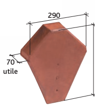
Fronton pour faitière angulaire à emboitement Réf. 801
