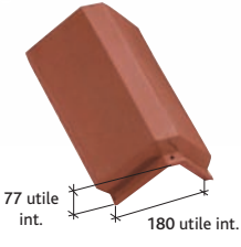
Faitière/arêtier angulaire à emboitement (3 au ml) Réf. 710 Crochet adapté : crochet F3-Réf. CRP 705
