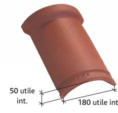
Faitière/arêtier 1/2 rond à emboitement petit modèle (3 au ml) Réf. 700 (1) Crochet adapté : crochet F6-Réf. CRP 700/706
