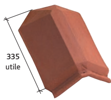
About d'arêtier angulaire à emboitement Réf. 859
